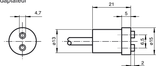
Adaptateur
