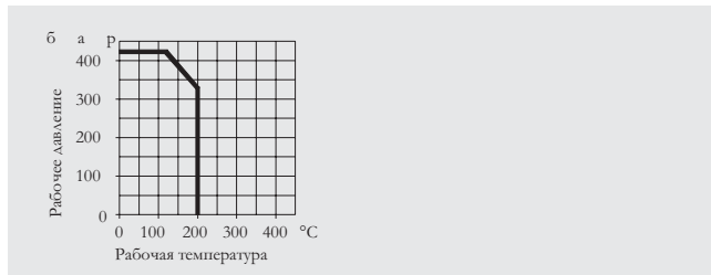
Доп. рабочее давление в зависимости от рабочей температуры
