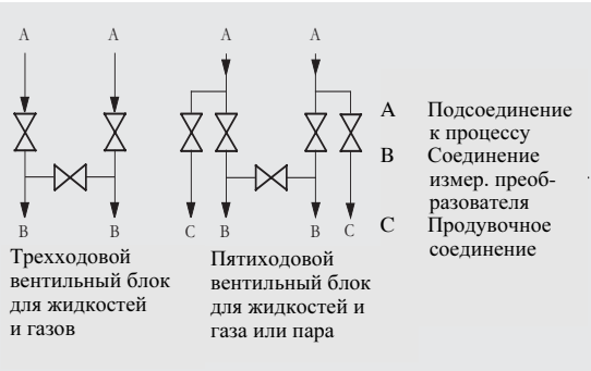
3-х и 5-ти ходовые вентильные блоки, схема
