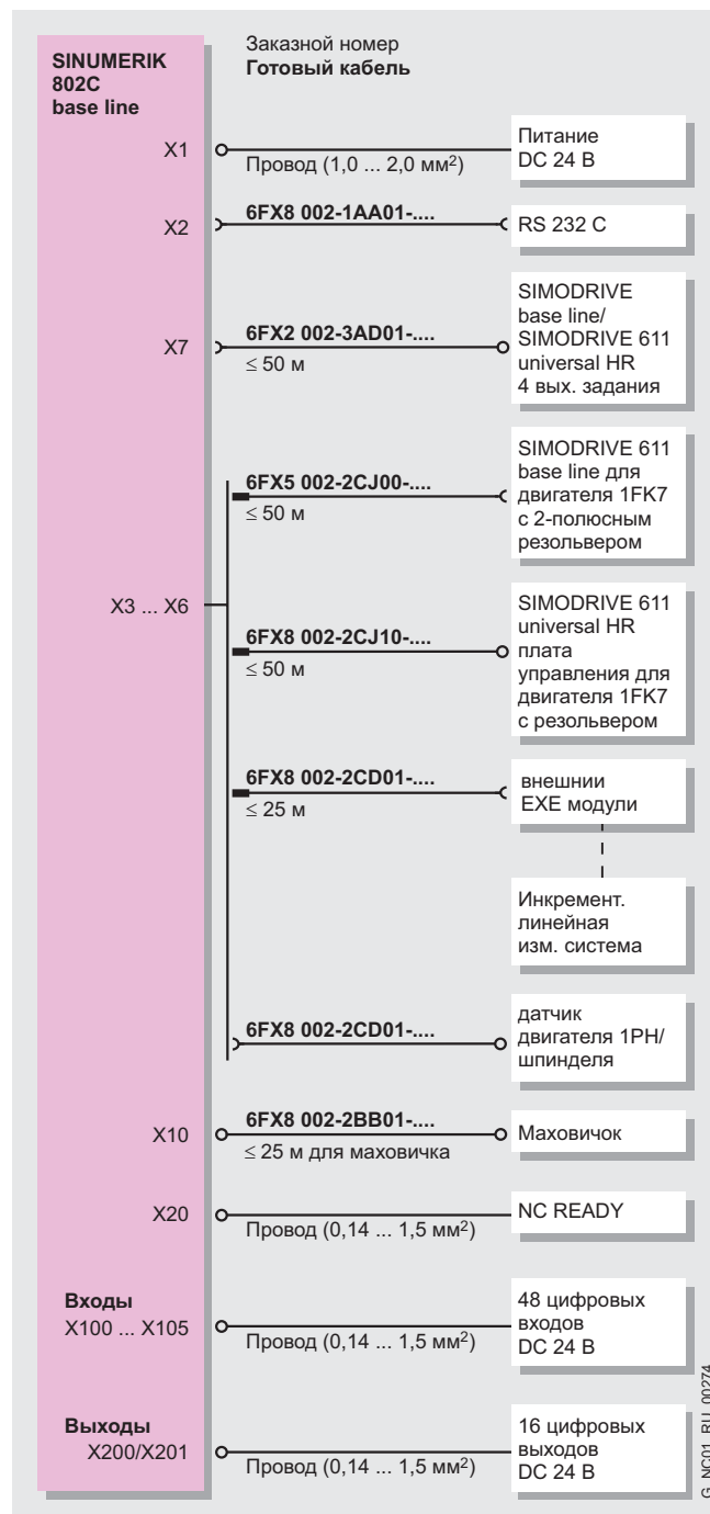
Обзор подключений SINUMERIK 802C base line
